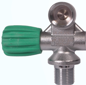
Mono valve M26 232 BAR M25x2 #N10048
