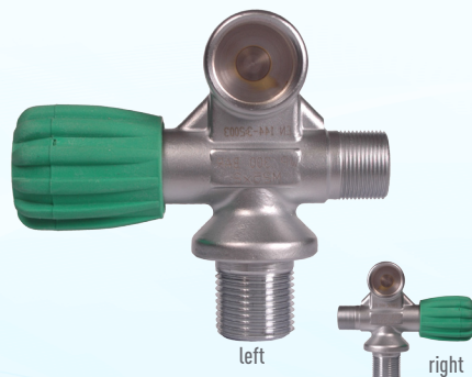
Modu valve M26 300 BAR M25x2 #N10155SD3 left #N10156DD3 right
